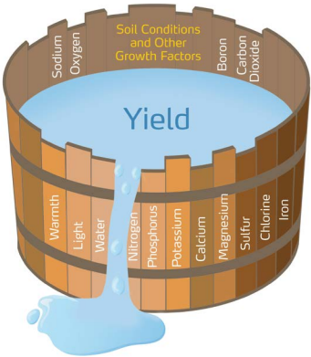
Liebig barrel
